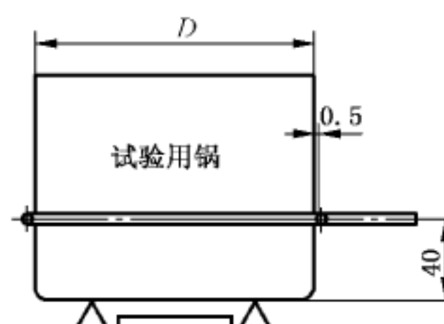
图 3 平底锅用取样器的安装位置
