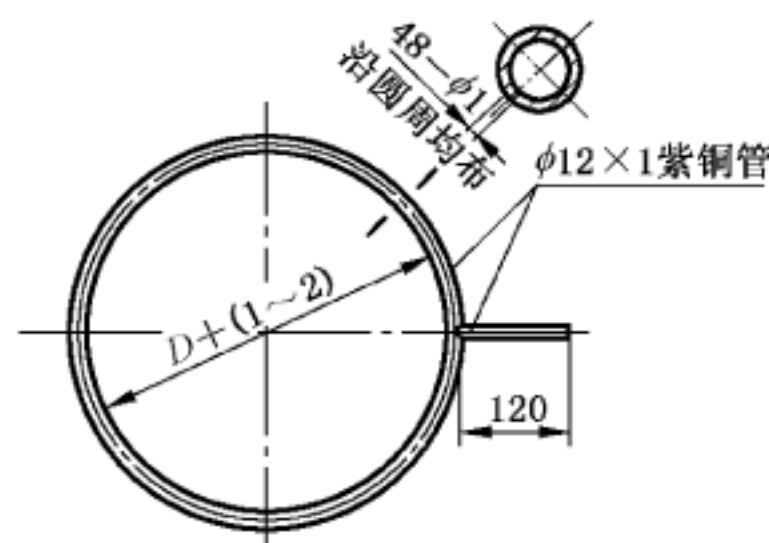
图 2 平底锅用取样器
