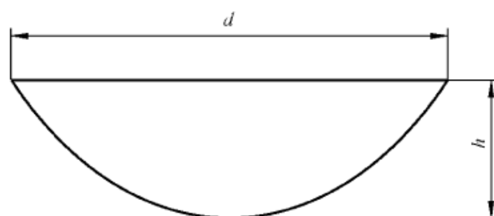
图 11 试验用锅结构尺寸
